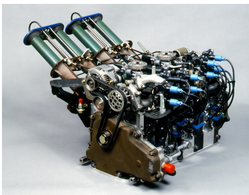
Il motore rotativo R26B a 4 rotori della Mazda 787B
